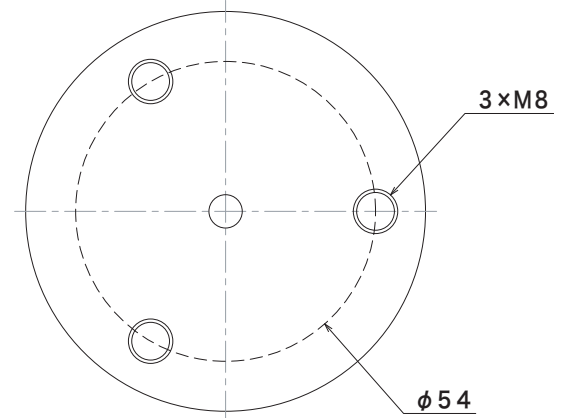
A矢视图
