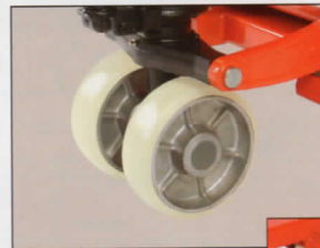
抗菌ホワイトウレタン車輪 (アルミ芯) ●標準タイプ(CP-10~20)に対応。
